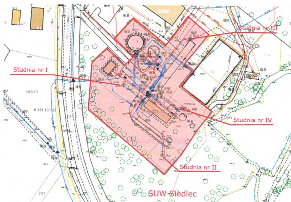
Plan sytuacyjny określający położenie studni I, II, III i IV na terenie SUW Siedlec.
